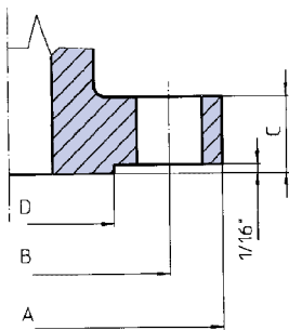
FLANGES ANSI - B16.5
